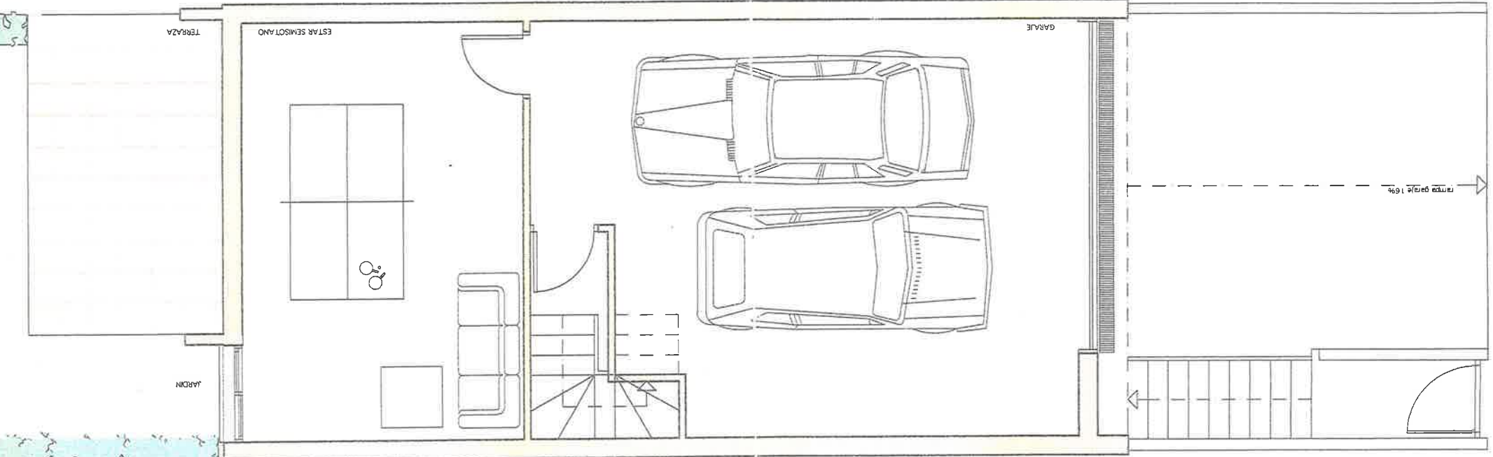
planta semisotano escala 1/50
